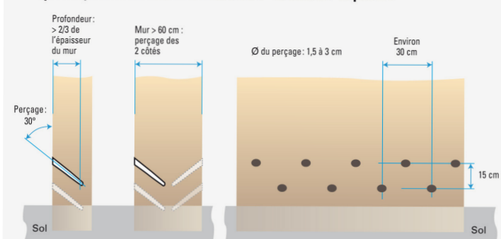
Principe d'injection du Minéralisant Guard® Remontée Capillaire
